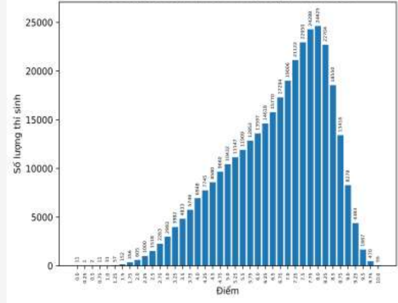
Biểu đồ phổ điểm thi THPT môn Vật lý - năm 2024
