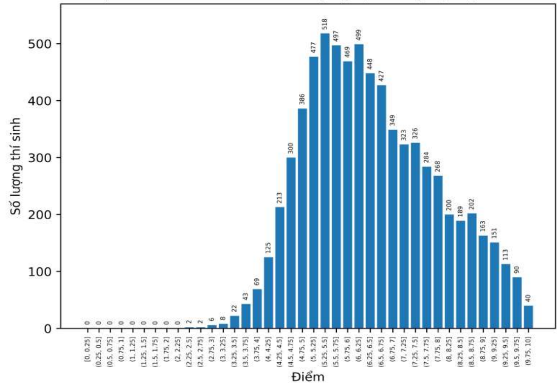
Biểu đồ phổ điểm thi THPT môn Công nghệ - Công nghiệp - năm 2026
