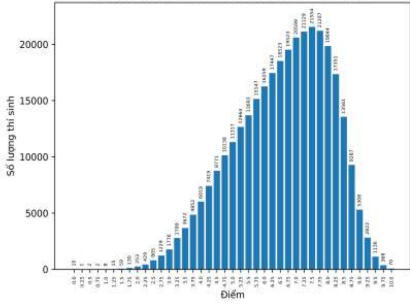
Biểu đồ phổ điểm thi THPT môn Vật lý - năm 2023
